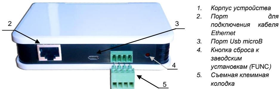
Рис. 1. Внешний вид ProxWay PW-A модификации 2
