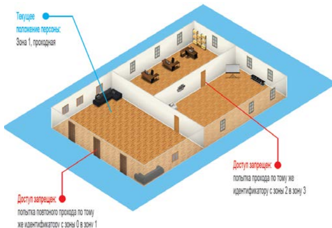
Рис 6. Отслеживание нарушений
