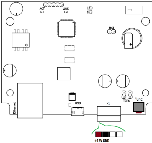
Рис. 2б. Внешний вид платы контроллера модификации 2
