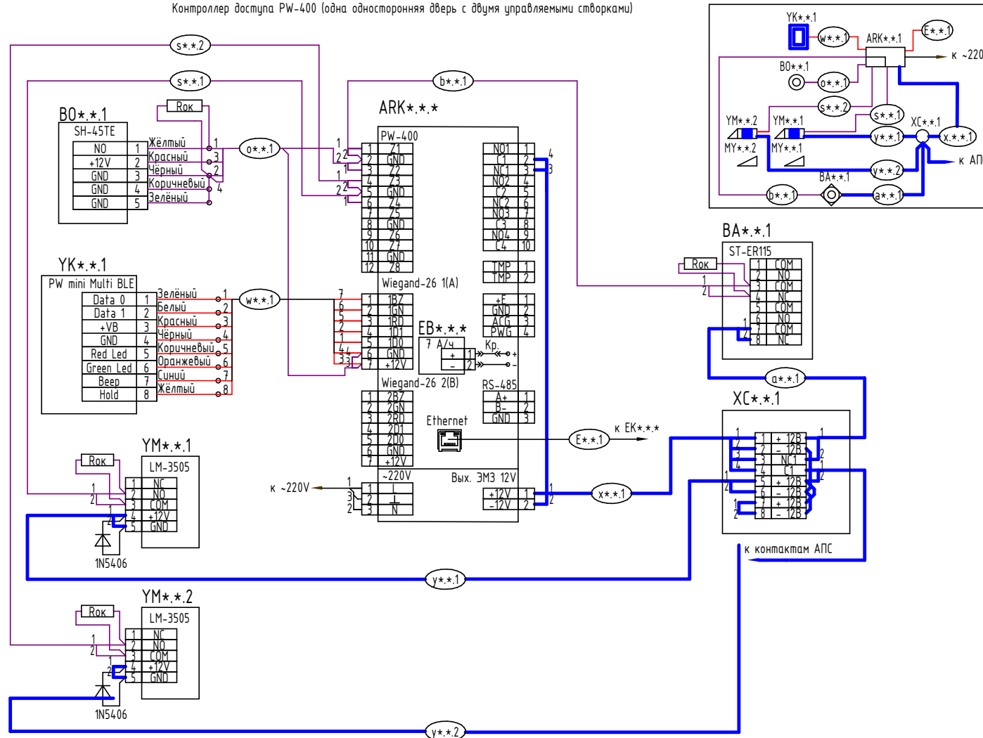
Схема электрическая, подключений, типовая. Контроллер доступа PW-400 (одна односторонняя дверь с двумя управляемыми створками)
