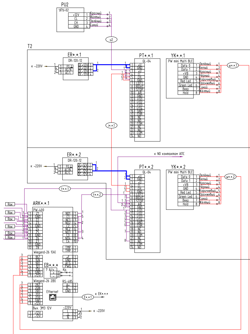
Схема электрическая, подключений, типовая. Контроллер доступа PW-400 (турникет QL-04 с пультом управления УПУ-02)
